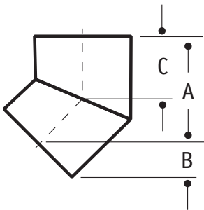
COUDE 60°
